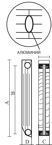
Чертежи радиатора в разрезе
